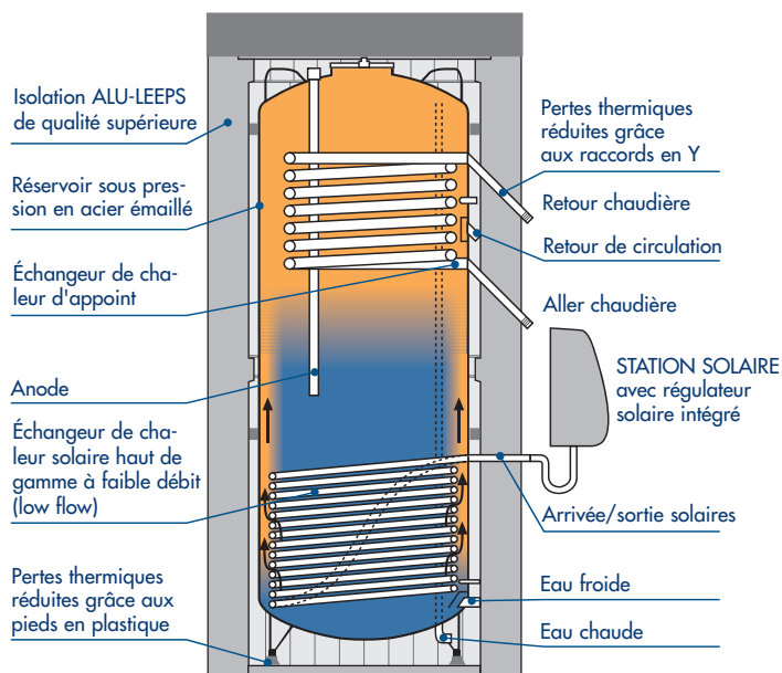
Coupe du COAX 390
